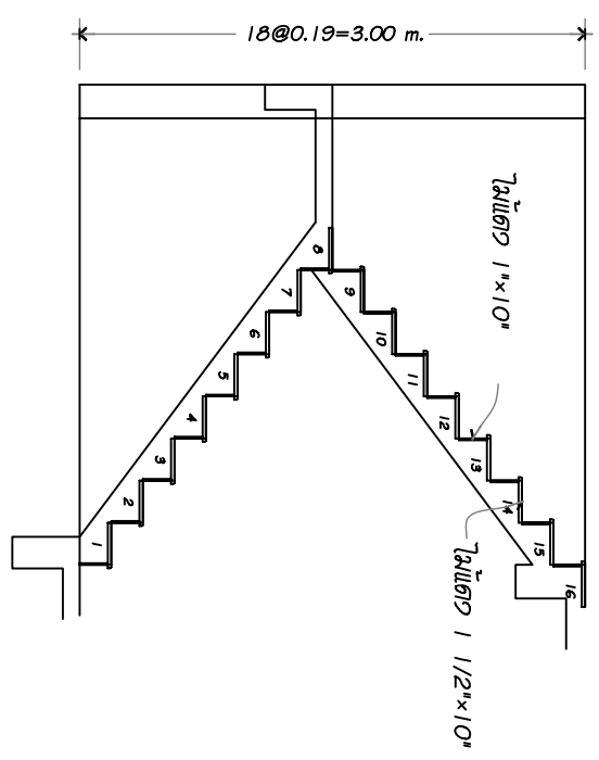
รายละเอียดบันได ST1 มาตราส่วน 1:50
