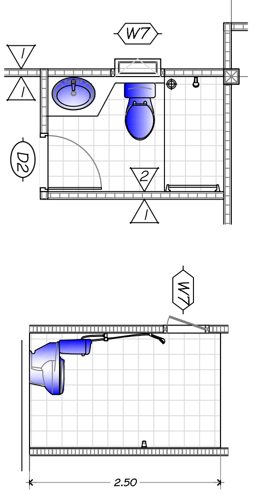
แปลนห้องน้ำ 1 มาตราส่วน 1:50
